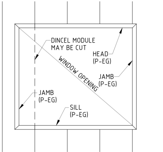
DINCEL WALL ELEVATION
